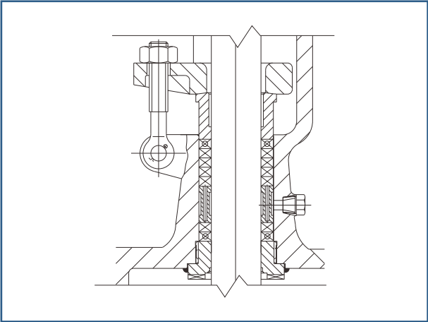
水封结构
