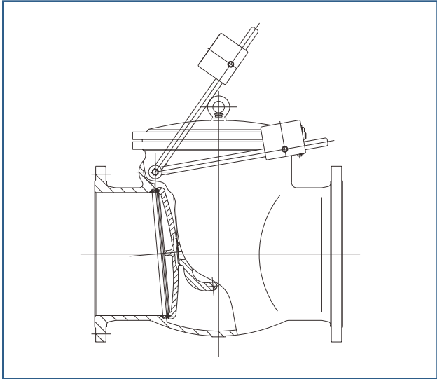
止回阀重锤设计
