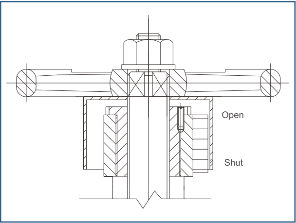
截止阀上的位置指示器
