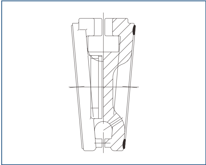
压力泄放孔
