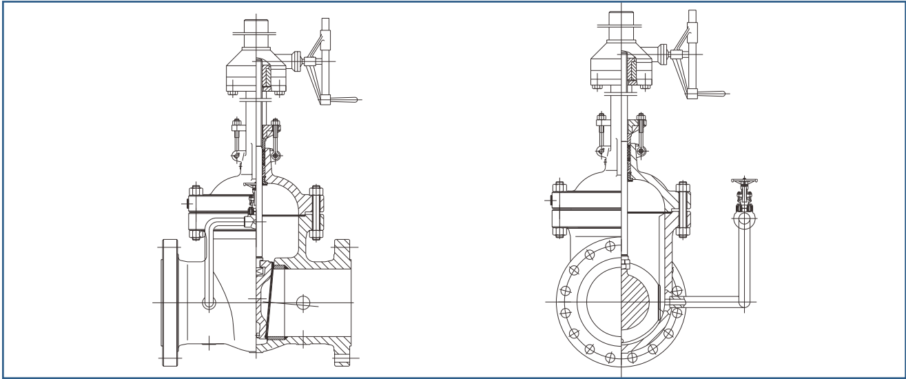
旁通结构
