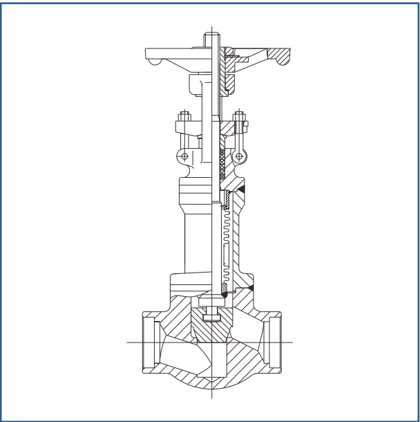
锻钢波纹管阀
